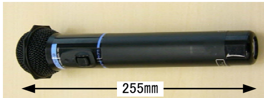
赤外線ワイヤレスマイク(ハンド型) ビクター WM-PH711/712/713/714
